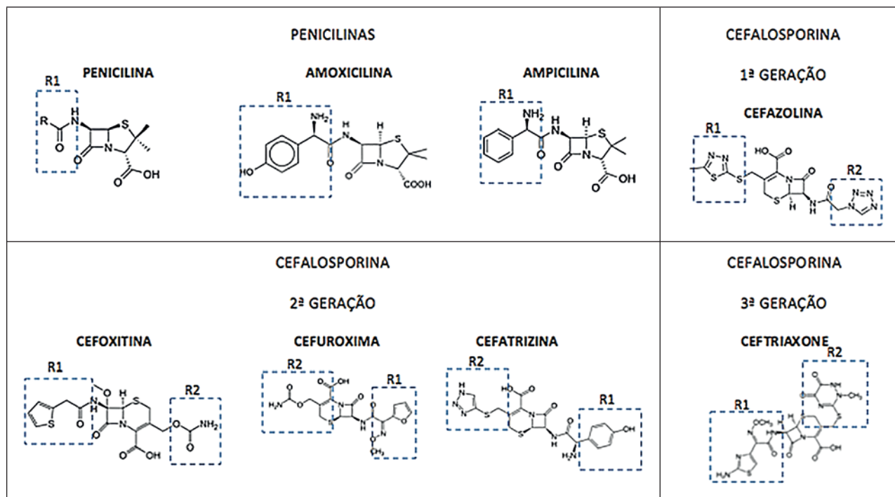
Figura 2. Estrutura química das penicilinas e algumas cefalosporinas
