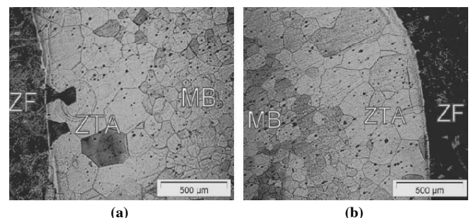
Fig. 2. Microestrutura da junta soldada com metal de adição: a) E316L e b) E309L. Ataque: Água Régia.
