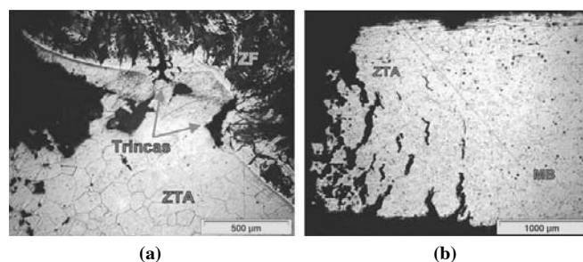
Fig. 6. Fissuras (trincas) de Corrosão sob tensão a) na zona de ligação da junta soldada com o metal de adição E309L e b) na ZTA da junta soldada com o metal de adição E316L. Microscopia Ótica. Ataque eletrolítico: Ácido Oxálico.
