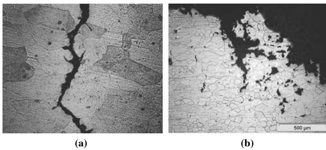
Fig. 7. Fissura: a) Intergranular de CST desenvolvida na junta soldada com o metal de adição E309L. Aumento: 200 x; b) Transgranulares de CST desenvolvida na junta soldada com o metal de adição E309L. Microscopia Ótica. Ataque eletrolítico: Ácido Oxálico.
