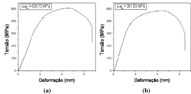
Fig. 4. Ensaio de tração mecânica realizados nas juntas soldadas com os metais de adição: a) E309L e b) E316L.
