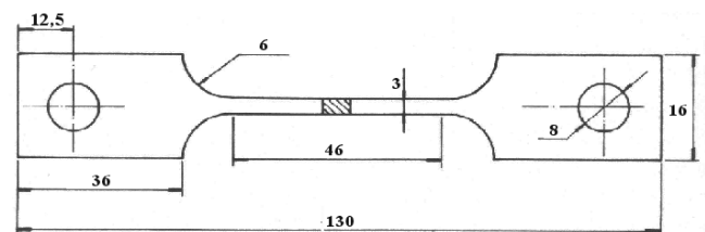
Fig. 1. Dimensões dos corpos de prova em milímetros.
