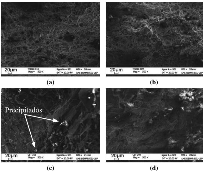
Fig. 8. Microfratografias de CPs ensaiados por: a) Tração Mecânica – Metal de adição E316L; b) Tração Mecânica – Metal de adição E309L; c) CST – Metal de adição E316L; d) CST – Metal de adição E309L.
