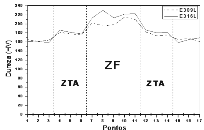
Fig. 5. Perfil de dureza do Aço AISI 444 soldado com os metais de adição E309L e E316L.
