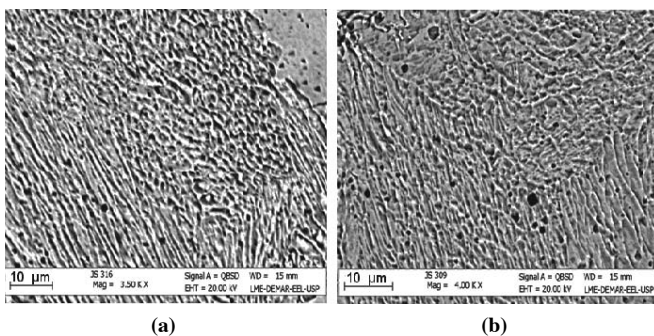
Fig. 3. Microestrutura da ZF com o metal de adição a) E316L e b) E309L. Ataque: Água Régia
